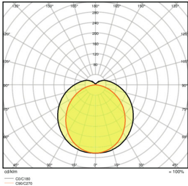
DP SLIM VALUE 1200 36 W 6500 K IP65 GY
